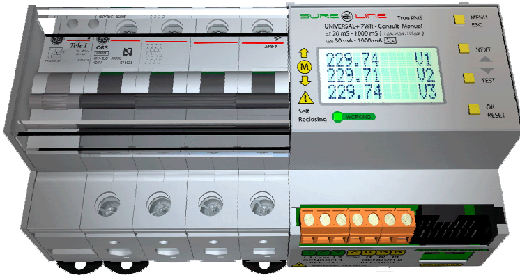
5PM+: MCB magnetotérmico de 6 a 63A, 2 y 4 polos, Icu 6-10Ka
