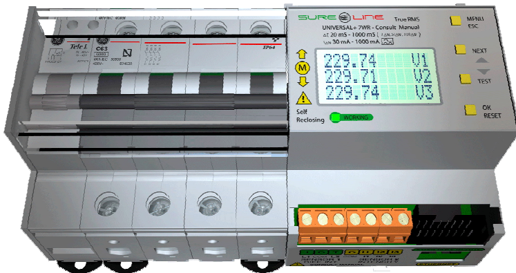
K+: MCB magnetotérmico de 6 a 63A, 2 y 4 polos, Icu 6-10Ka
